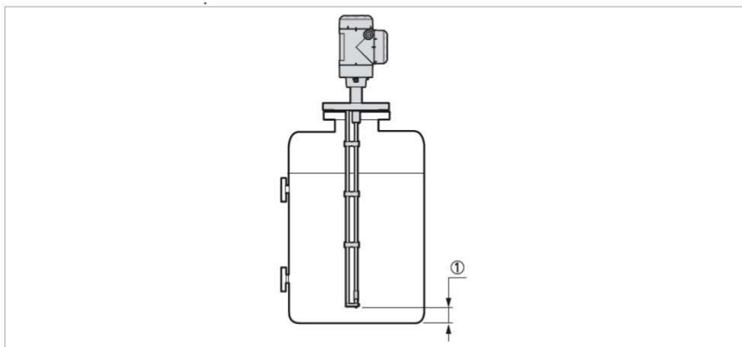
图 8-19: 安装反向界面天线的最小限度
