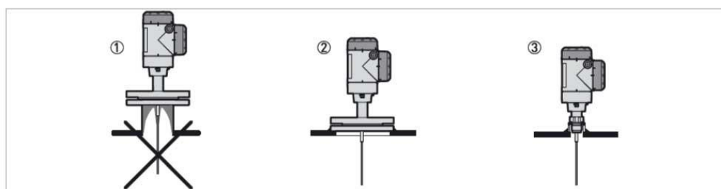
图 8-15：如何防止所测介质在过程连接件四周的堆积问题
