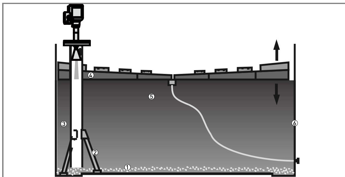
图 8-11: 浮顶
