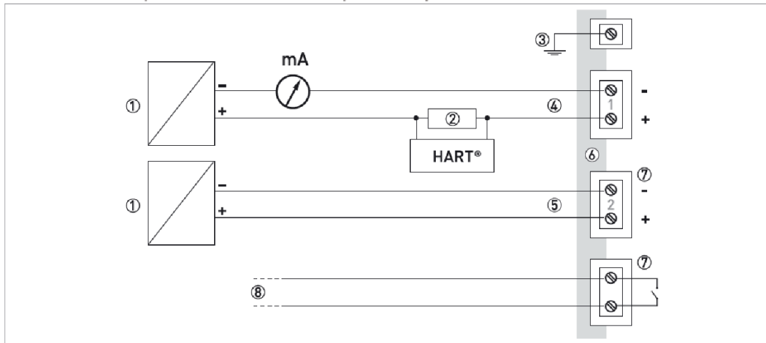
图 5-7: 1 个电流输出和 1 个开关量输出-继电器
