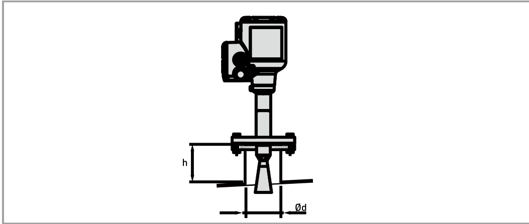
图 8-6: 法兰连接
