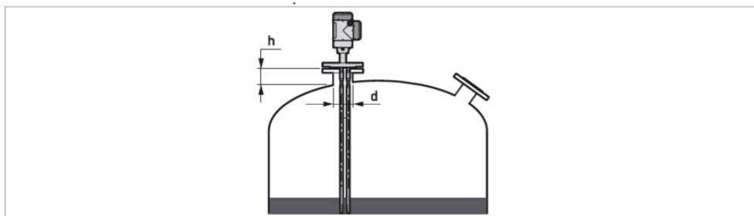
图 8-18: 双杆和双缆天线的推荐短脖尺寸
