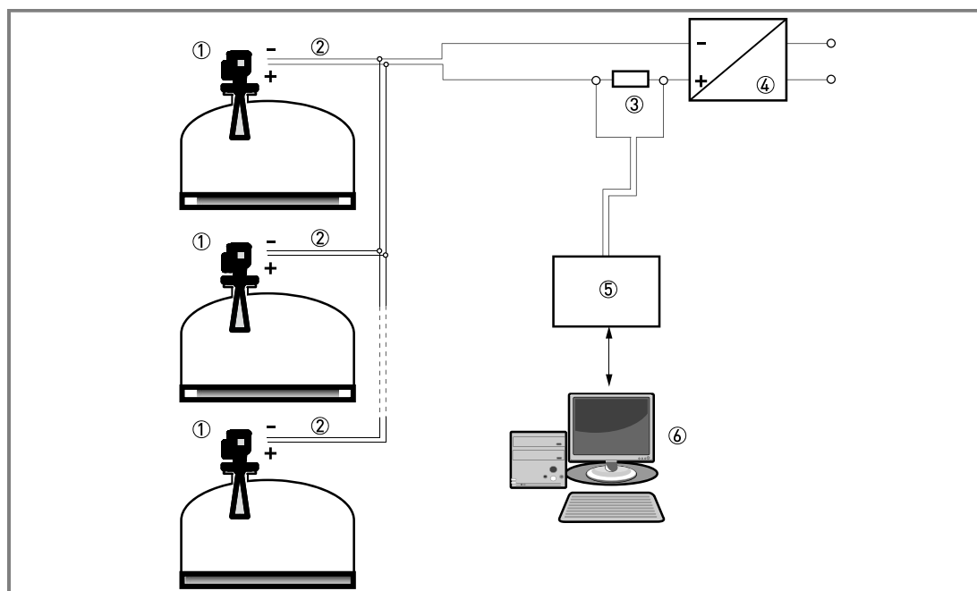
图 6-2: 多点网络
