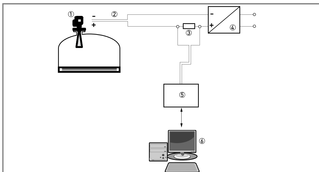
图 6-1: 点对点连接
