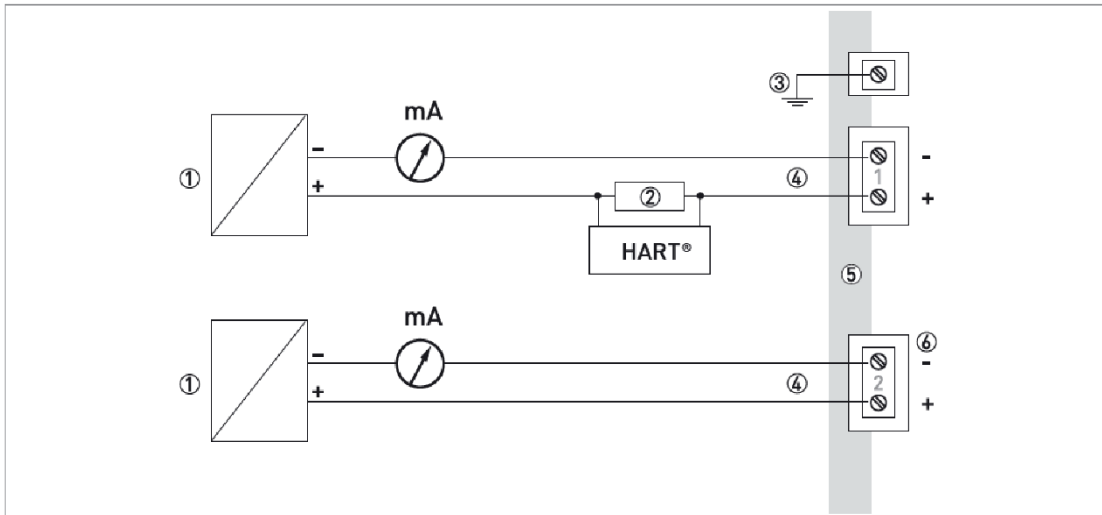
图 5-6:非防爆型仪表的电气连接件 (2 个电流输出)
