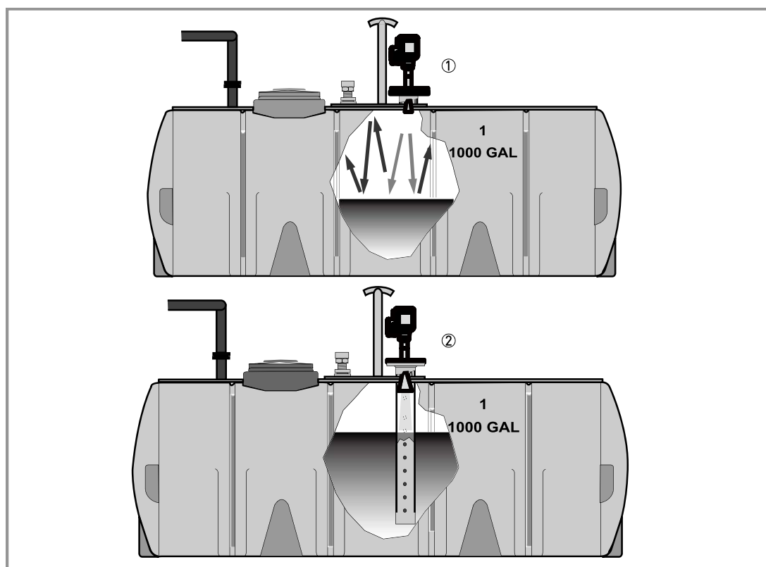
图 8-12: 水平卧罐
