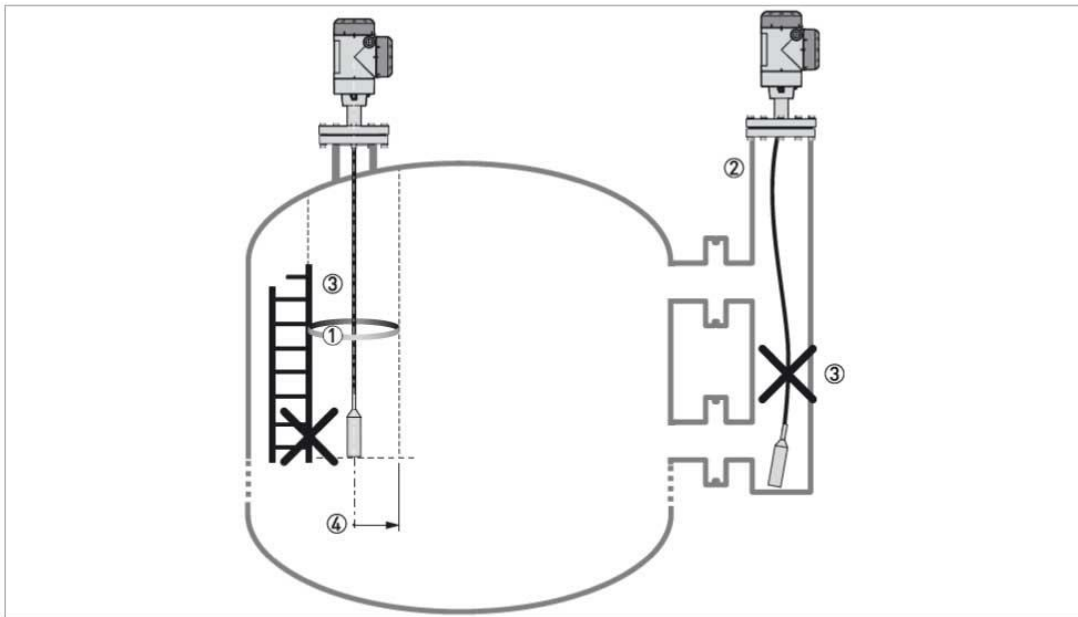
图 8-20: 液体测量的安装建议
