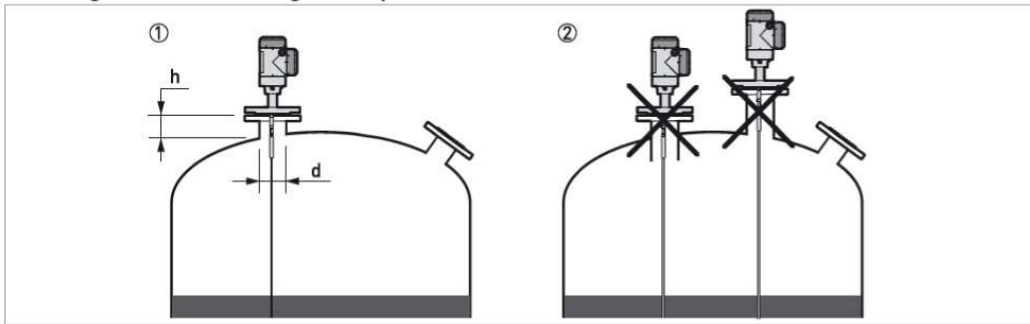
图 8-16: 单杆和单缆天线的推荐短脖尺寸
