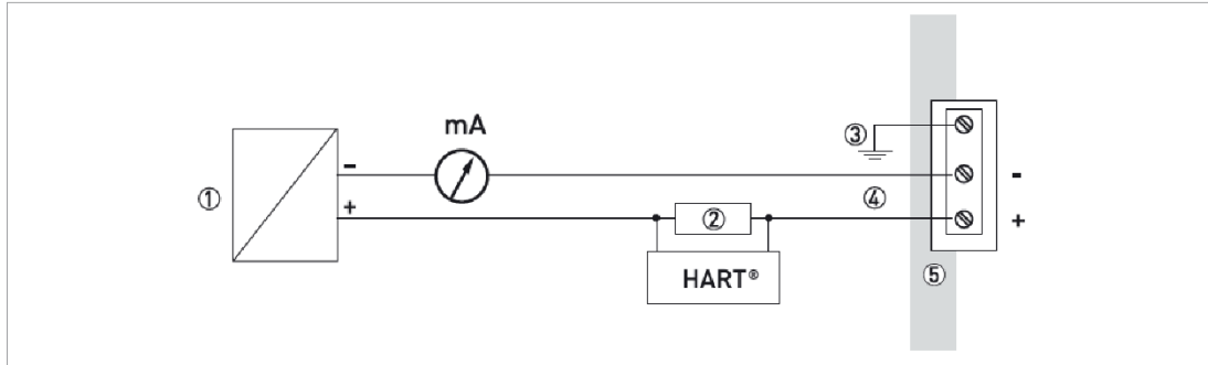
图 5-5:非防爆型仪表的电气连接件 (1 个电流输出)
