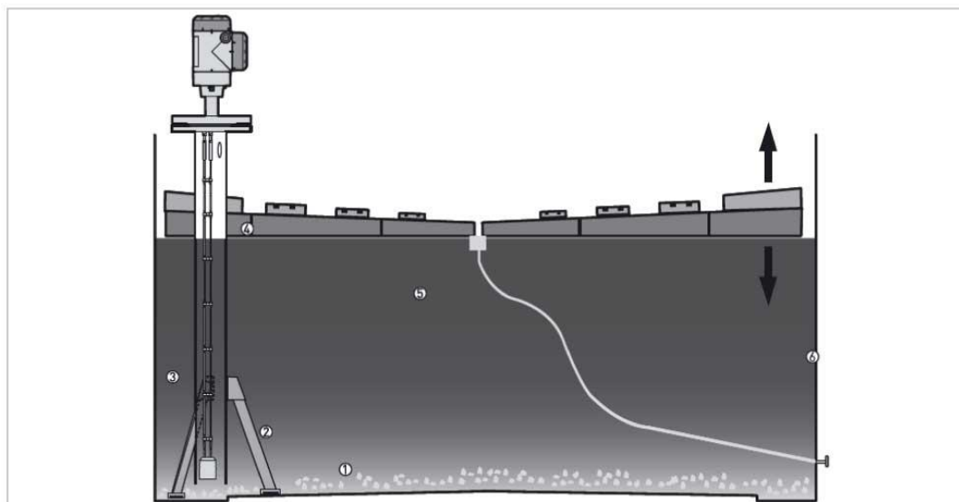
图 8-22: 浮顶
