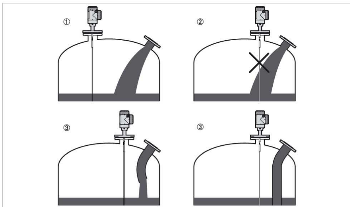
图 8-14：请勿将设备放在介质入口附近。
