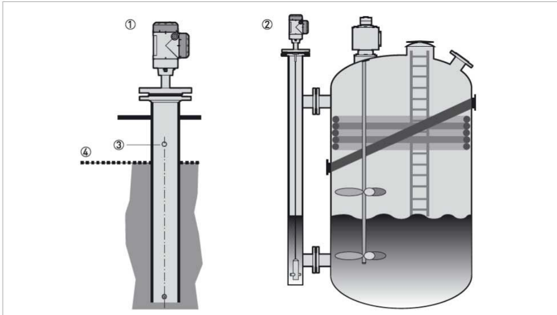
图 8-21: 立管（导波管和旁通管）安装建议
