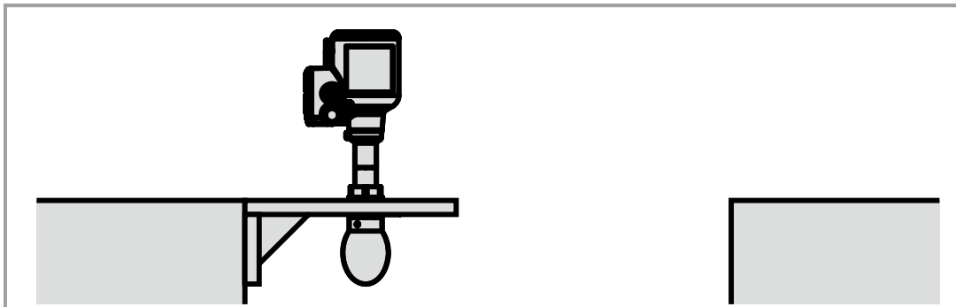
图 8-9: 敞口井坑
